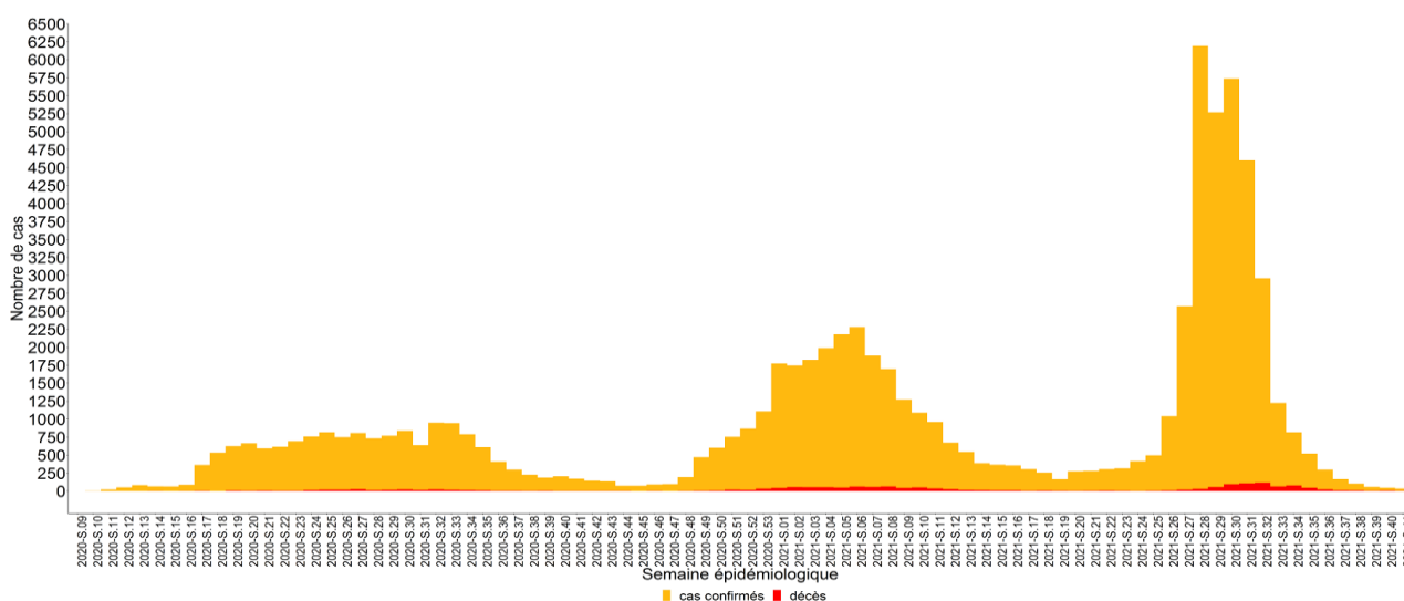
Graphique 2 : Courbe hebdomadaire des cas confirmés et des décès de COVID-19 du 02 mars 2020 au 18 octobre 2021, Sénégal
